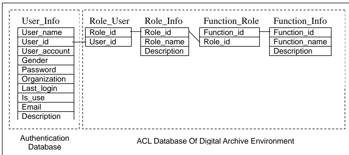
圖6：權限管理系統資料庫設計
