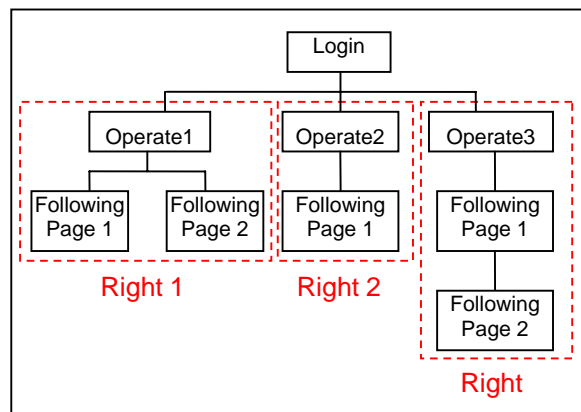
圖4：網頁與權限隸屬關係圖
