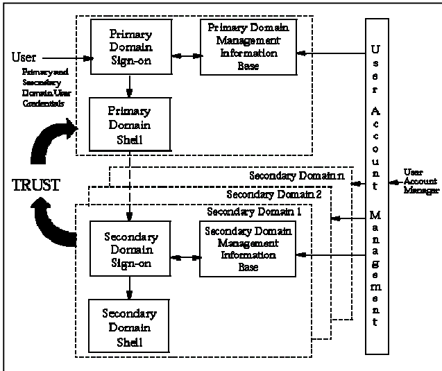
圖2：SSO示意圖[5]
